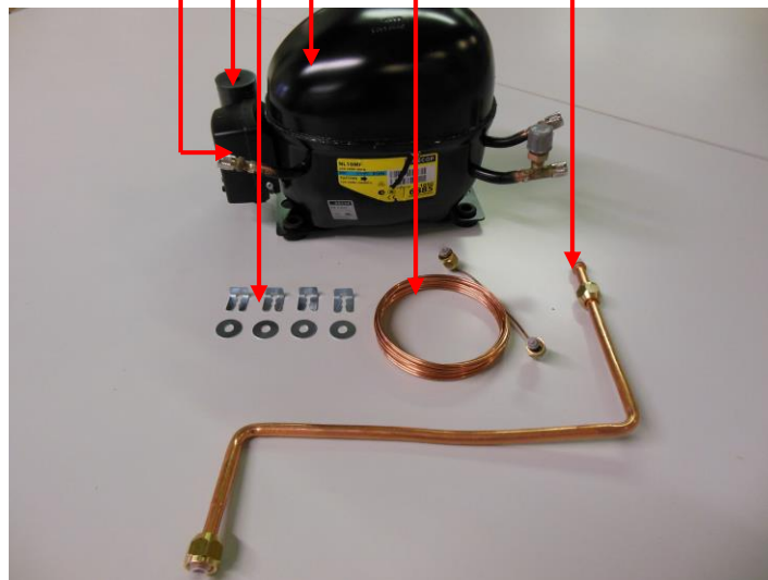
Ersatzkompressor ASC (Set) Art.Nr.: 4440100015
