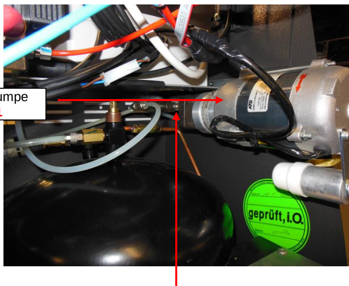
Zubehör Elektro-Innenzahnradpumpe Art.Nr.: 4441600099
