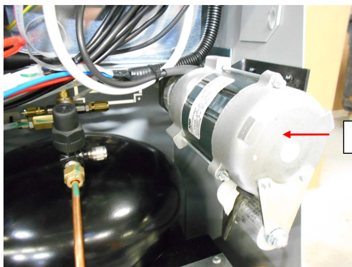
Elektro-Innenzahnradpumpe Art.Nr.: 4441600091
