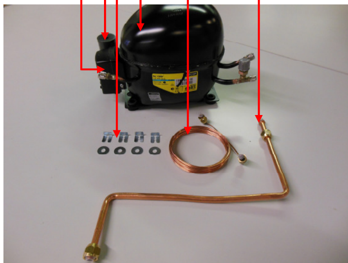
Ersatzkompressor ASC Art.Nr.: 4440100015
