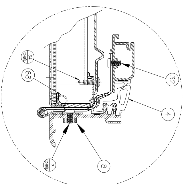
SECTION B-B SCALE: FULL
