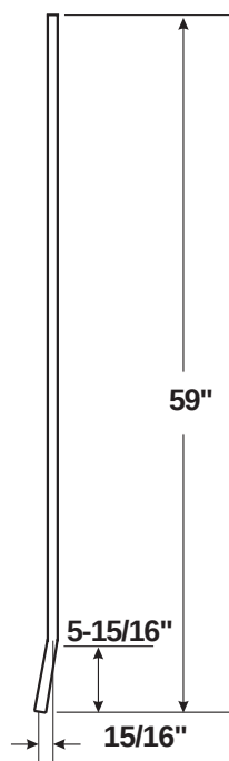
LH Arm
