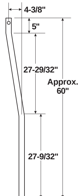
RH Arm
