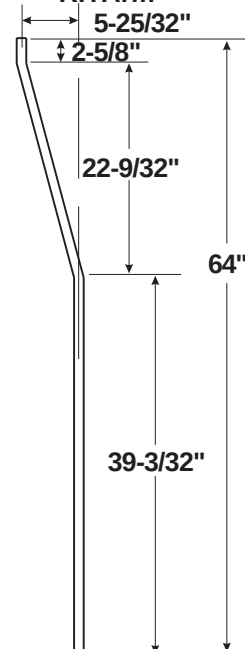
RH Arm
