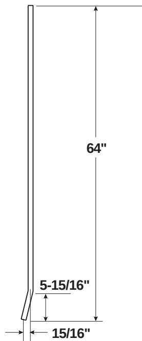
LH Arm
