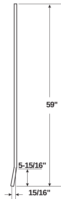
RH Arm
