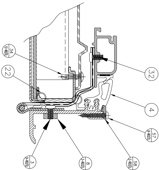
SECTION B-B SCALE: FULL
